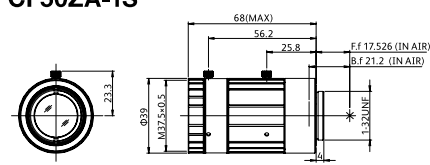
CF50ZA-1S
