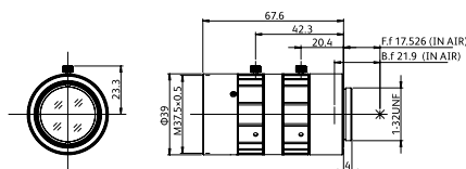
CF12ZA-1S
