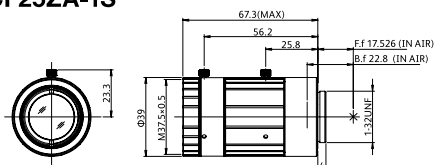
CF25ZA-1S
